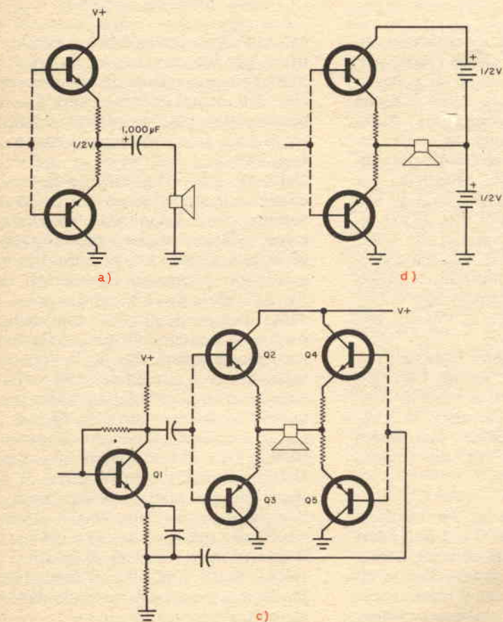
Fig. 1 - Circuiti basilari OTL (a) e OCL (b). Il circuito (c) è quello di un amplificatore amplificato OTL/OCL di tipo a ponte.
