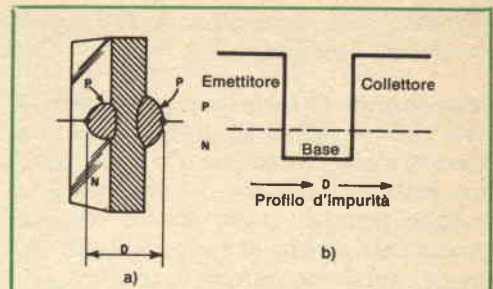
Fig. 11 - Tipico transistoro a lega.
