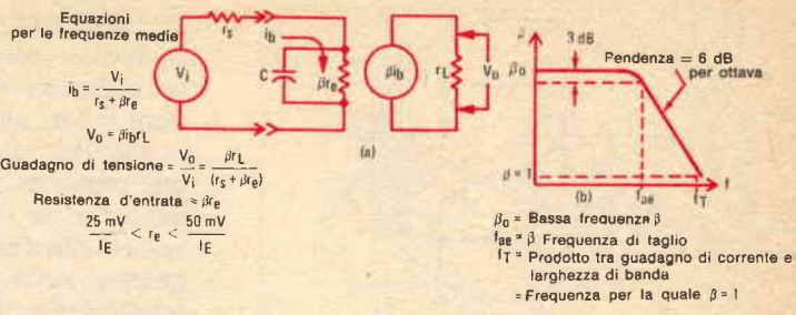
Fig. 7 - Circuito equivalente ad emettitore comune (a) e suo responso (b).
