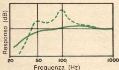
Fig. 3 - Condizioni di massima efficienza ai bassi (accompagnate però da marcati picchi nella curva di risposta) possono, nell'ascolto, far apparire ridotti i bassi profondi.
