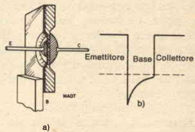
Fig. 13 - Tipo di transistoro a microlega diffuso.
