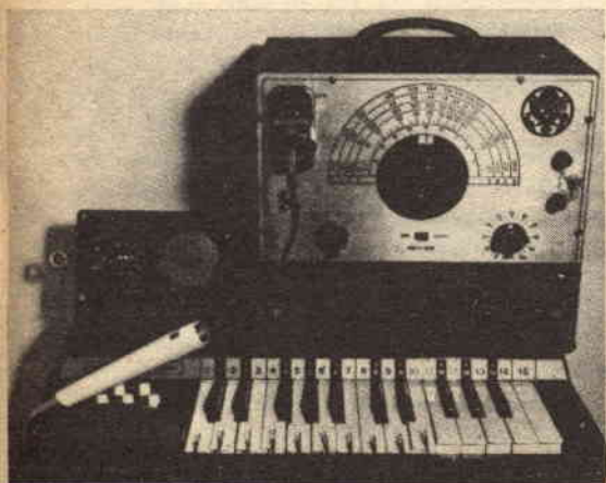
Fig. 5 - Dispositivo per effetti speciali per un organo elettronico; a destra sono montati il generatore audio e la tastiera, mentre i controlli per il sincronizzatore di cadenza, il miscelatore ed il microfono sono a sinistra.
