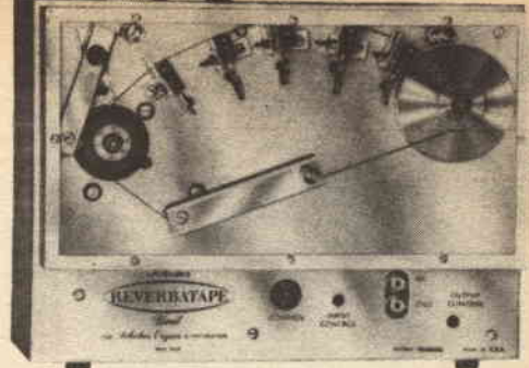
Fig. 3 - Questa unità Riverbatape della ditta Schober impiega un certo numero di testine ripetitrici.
